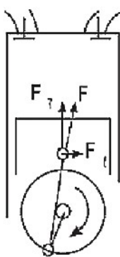
مکش
