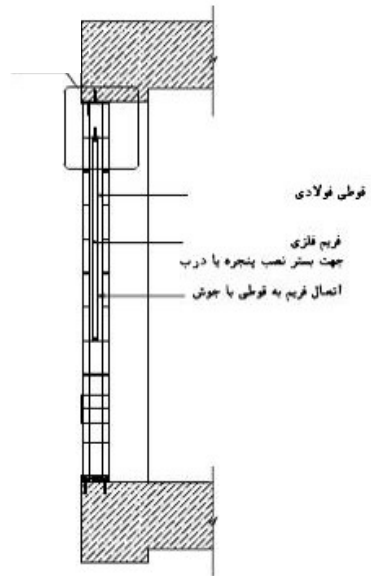
برش A-A
