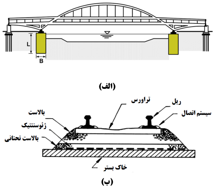
شکل ۴-۱ فونداسیون سازه های مختلف (الف) پل قوسی (ب) فونداسیون راه آهن (پ) فونداسیون آسانخراش های پتروناس
