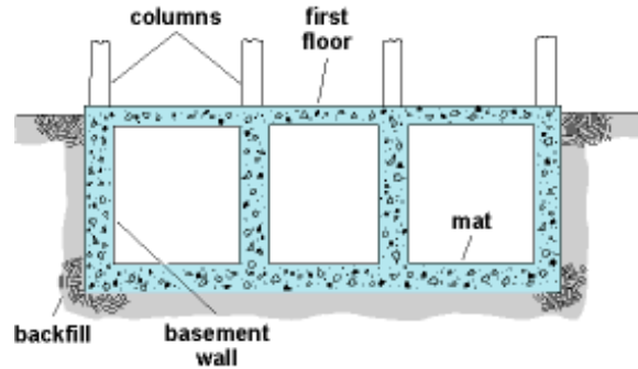
شکل ۲۰-۱ فونداسیون شناور
