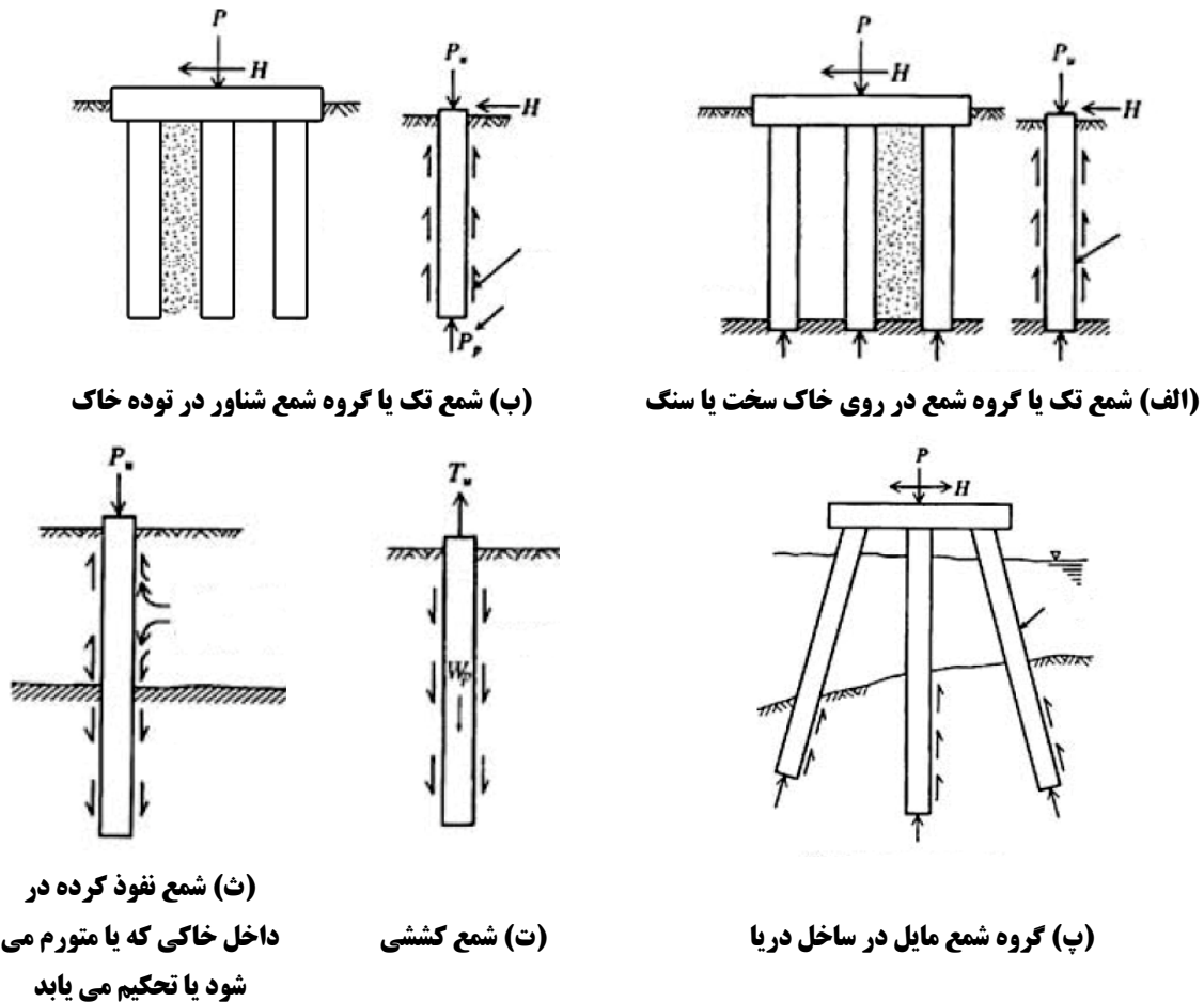
شکل ۱-۱۷ آرایش معمول شمع ها
