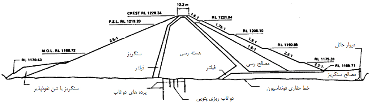
شکل ۳-۱ فونداسیون سد خاکی
