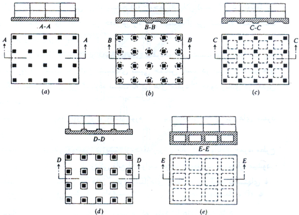
شکل ۱۵-۱ انواع مختلف فونداسیون های گسترده (a) سیستم دال تخت (b) سیستم قارچی (در بالا یا پایین) (c) سیستم دال دیوار (دال کف، دال سقف و دیوارهای میانی و جانبی) (d) سیستم جعبه ای
