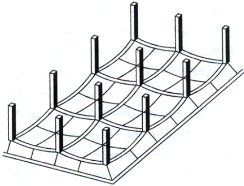
شکل ۲۱-۱ فونداسیون پوسته ای
