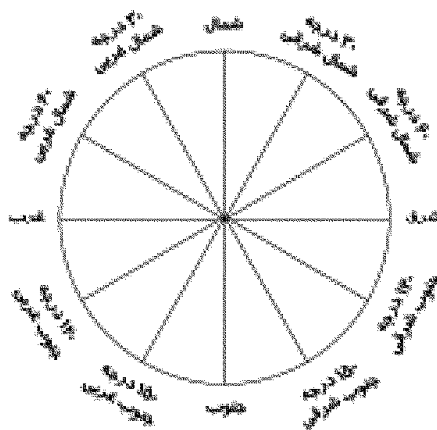
جهت‌گیری پنجره
